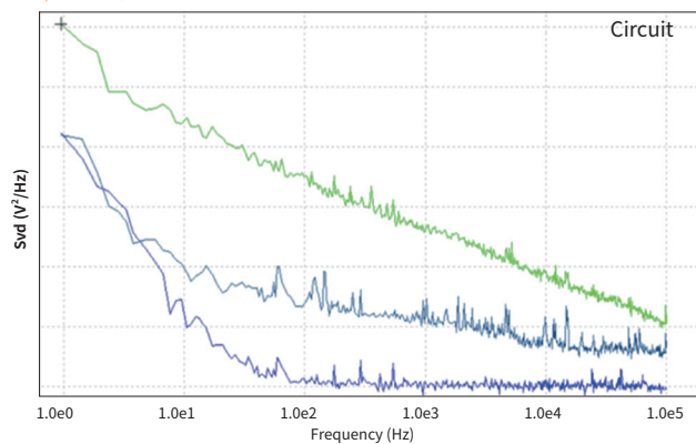
1/f 噪声测试, 电压功率谱
