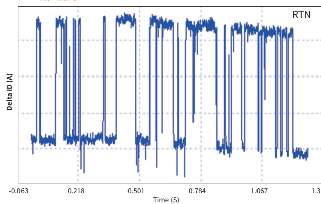
RTN 噪声测试
