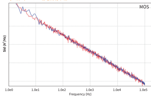
1/f 噪声, Drain 端电流功率谱
